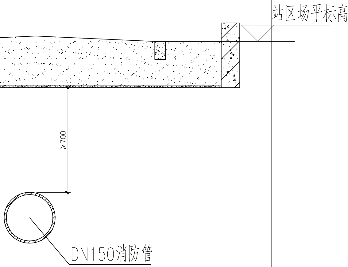
消防管与马路位置关系图
