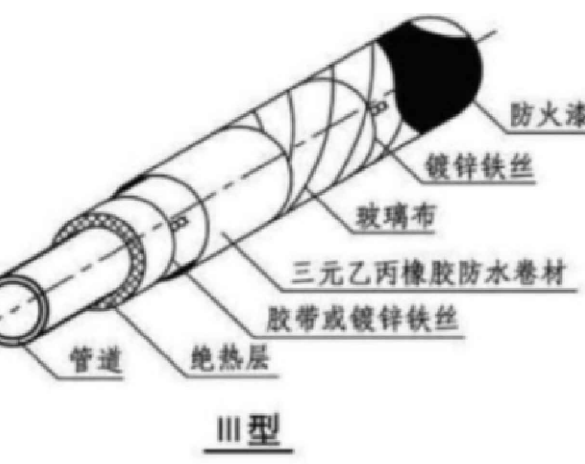
覆土内消防管保温做法示意图
