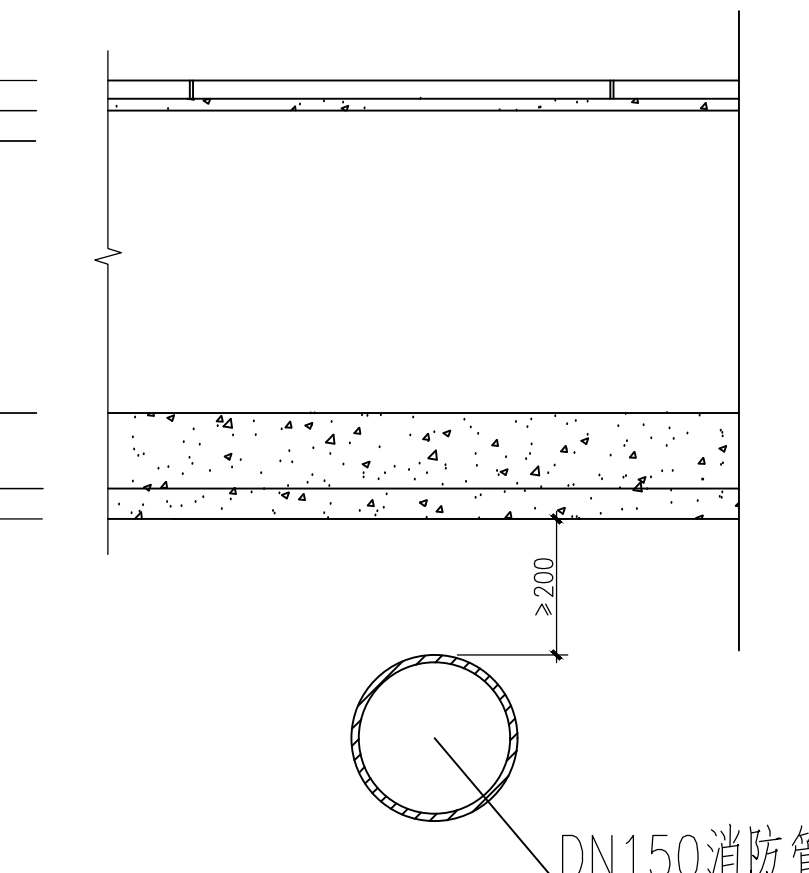
消防管与道路外电缆沟位置关系图
