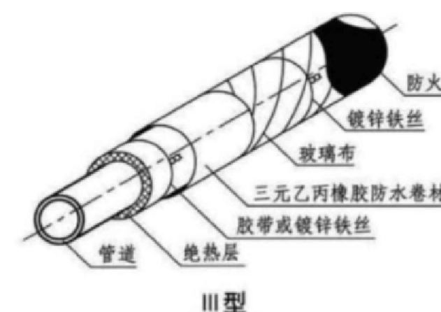
覆土内给水管保温做法示意图
